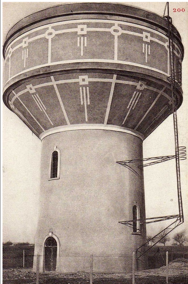
1928. - SOCIÉTÉ LYONNAISE DES EAUX ET DE L'ÉCLAIRAGE Réservoir en ciment armé de 700 m 3 sur tour de 11 mètres de hauteur, à Montataire, près Creil (Oise) Constructeur : Le Ciment Armé Demay Frères, à Reims
